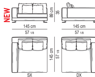
SOFÀ-ISOLA CHAISE LONGUE SOFÀ-CHAISE-LONGUE ISLE
