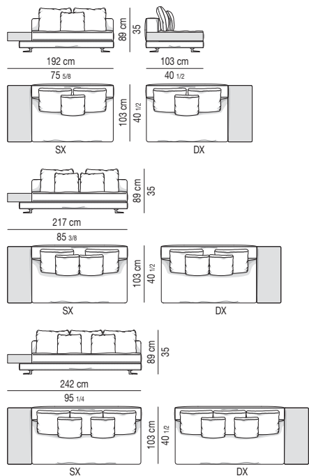
SOFÀ CON TOP 44X103 | SOFÀ WITH TOP CM 44X103
