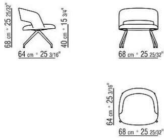
COD. 029837 ARMCHAIR CANALETTO / OAK / WENGE
